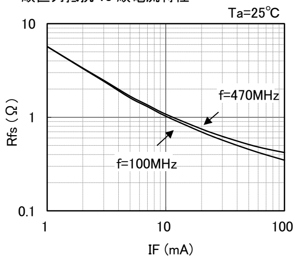
順直列抵抗 vs 順電流特性
