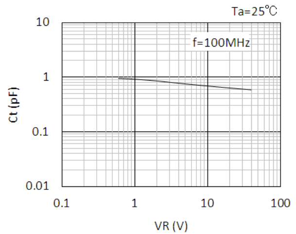
端子間容量 vs. 逆電圧特性
