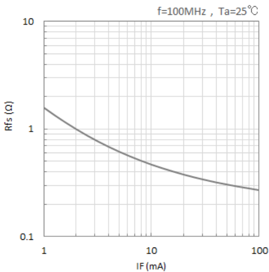
順直列抵抗 vs. 順電流特性
