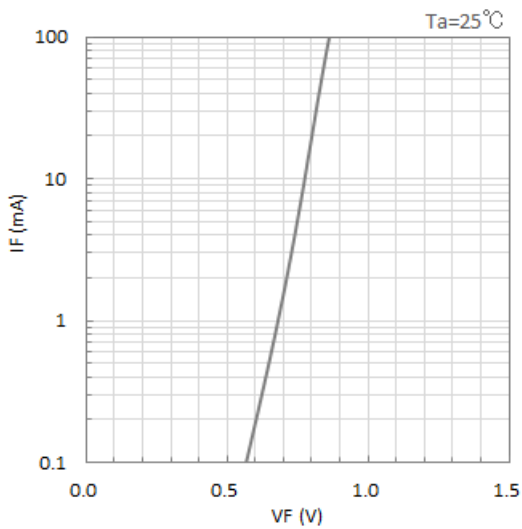
順電流 vs. 順電圧特性
